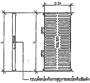
แปลนวางระบายน้ำรูปตัวยู ค.ส.ล. + ฝาดูแรงเหล็กหล่อระบายน้ำ มาตราส่วน NTS
