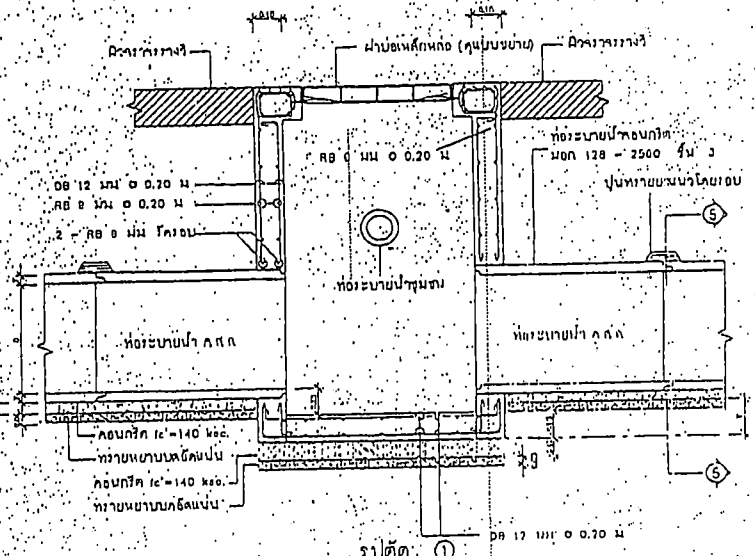
รูปตัด ① หน้ากว้าง 1 : 20
