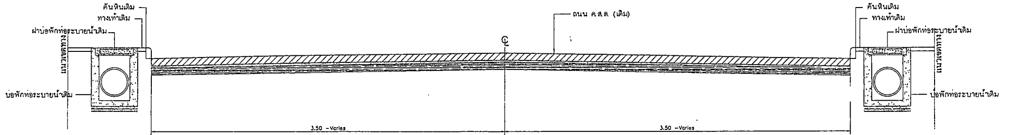
รูปตัด 2 (เก่า)
