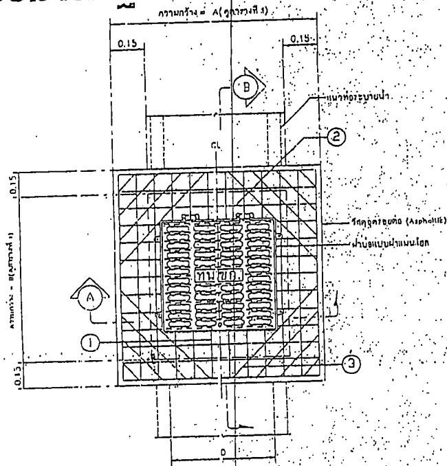
แปลนเหล็กเสริมโครงสร้างฉีดผ้าเบ้าเหล็กหล่อเหนียว NOT TO SCALE
