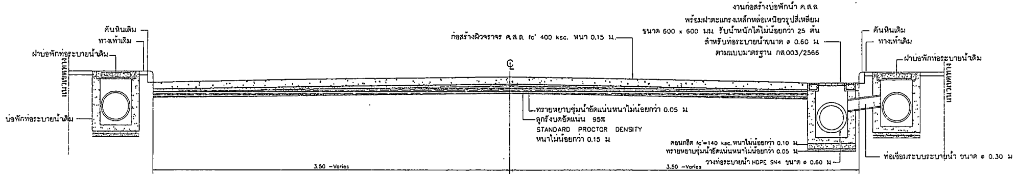
รูปตัด 2 (ใหม่)
