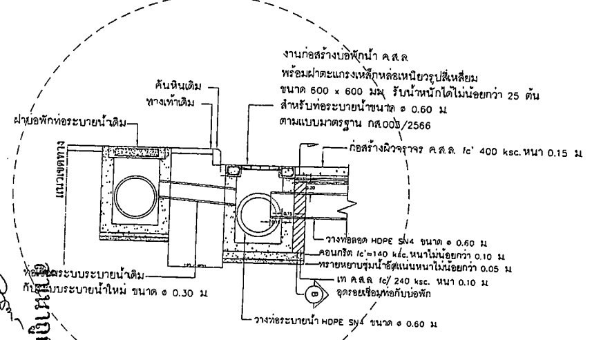
รูปตัด B NOT TO SCALE
