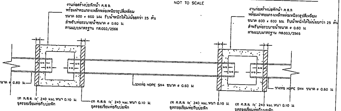
รูปตัด A NOT TO SCALE
