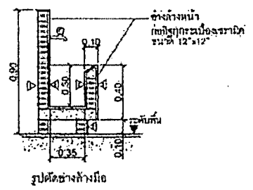
แบบขยายอ่างล้างมือ มาตราส่วน NTS
