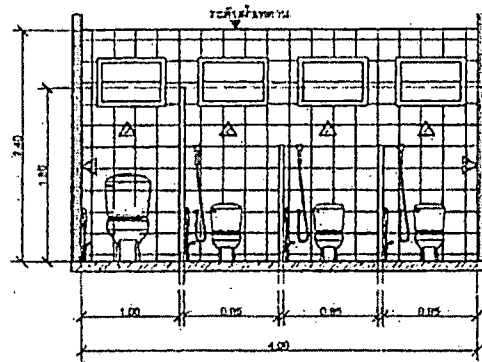
รูปตัด B-02
