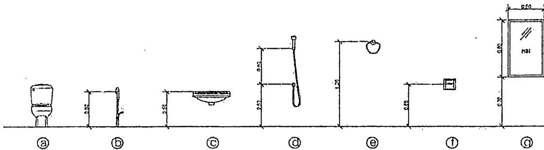
แบบมาตรฐานการติดตั้งสุขภัณฑ์
