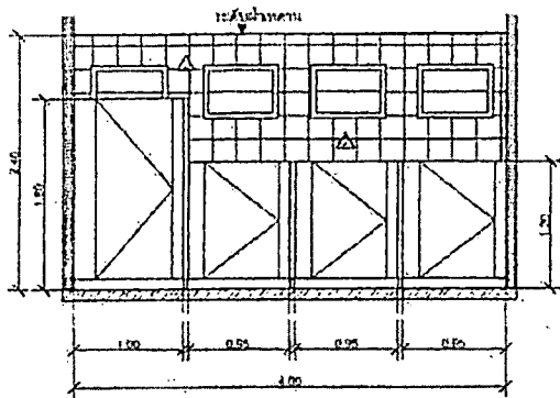
รูปตัด A-01
