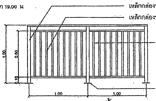
แบบขยายรั้ว มาตราส่วน NTS
