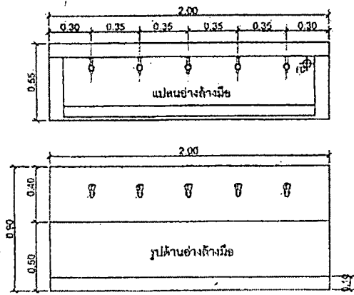
แบบขยายอ่างล้างมือ มาตราส่วน NTS
