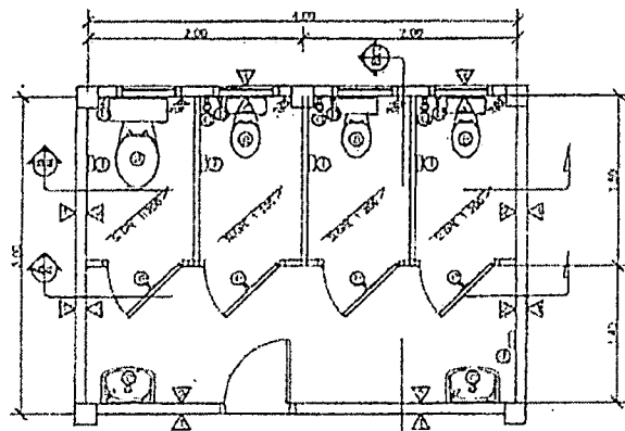
แปลนห้องน้ำ
