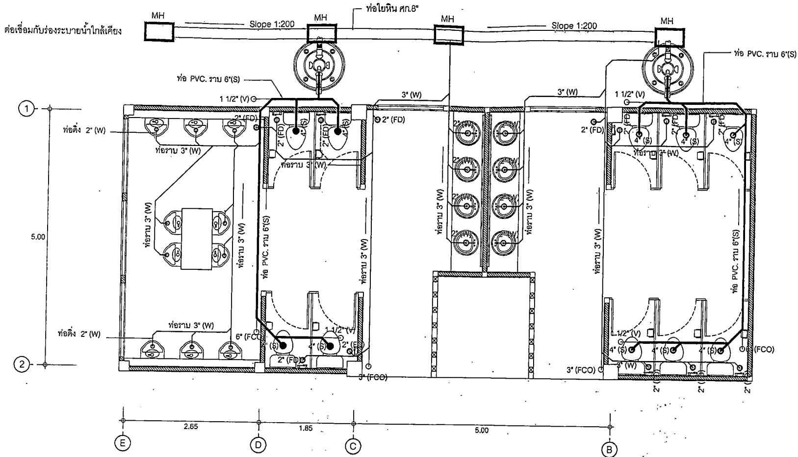
ผังระบบสุขาภิบาล
