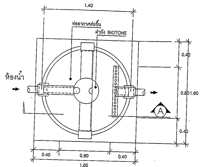
แปลนขยายถัง Biotone AP - 2000 Lt
