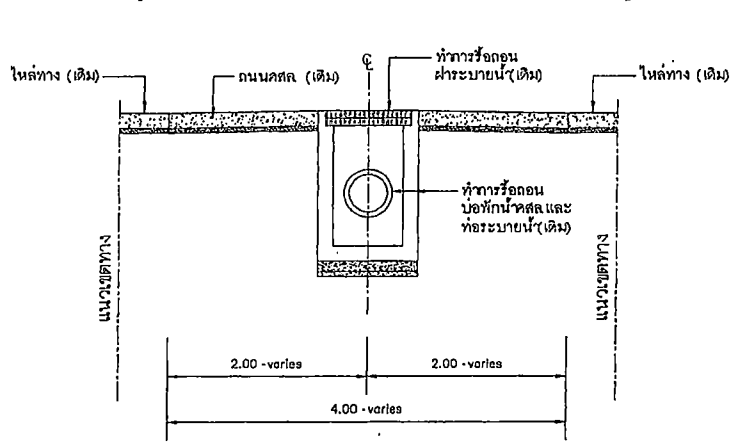
รูปตัด 2(เก่า) NOT TO SCALE
