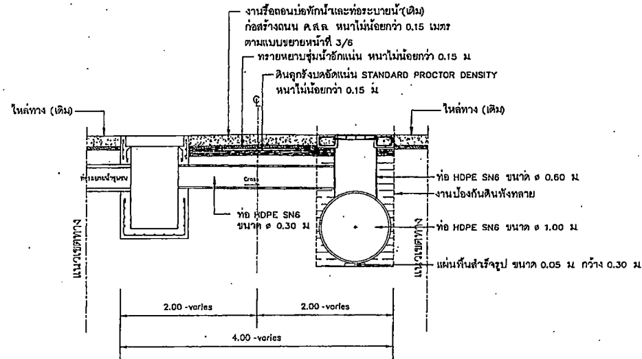
รูปตัด 2(ใหม่) NOT TO SCALE
