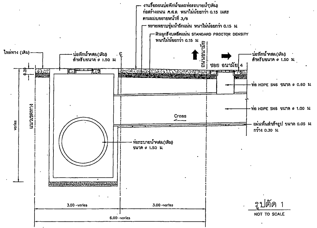
ตารางแสดงค่าระดับและระยะทาง จาก sta. 0+000 ถึง sta. 0+307 สำหรับ โครงกวดสร้างท่อระบายน้ำ รอยอนามัย 4 (ชุมชนโนนพัน)
