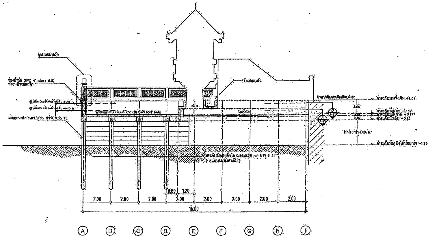
รูปตัด B - B SCALE 1 : 100
