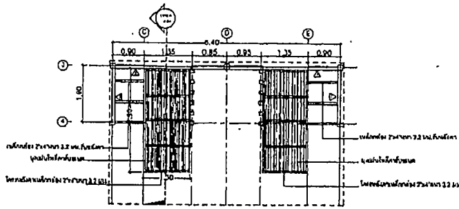
Section 3 มาตราส่วน 1:100
