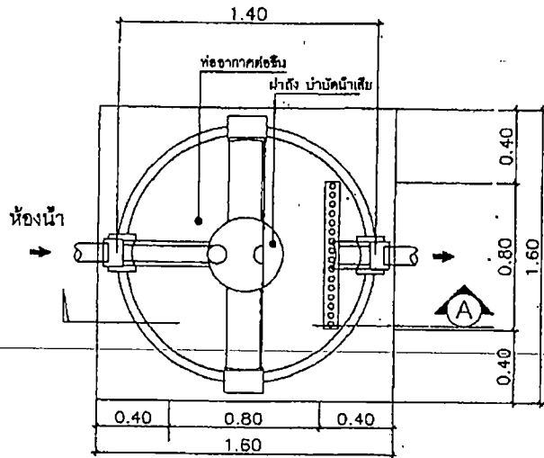
แปลนขยายถึง บำบัดน้ำเสีย
