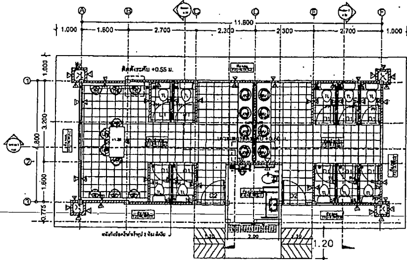
แปลนห้องน้ำ มาตราส่วน 1:100
