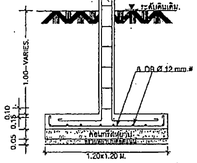
ขยายปรัด A-A มาตราส่วน 1:20
