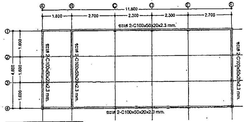
แปลนอะเส มาตราส่วน 1:50
