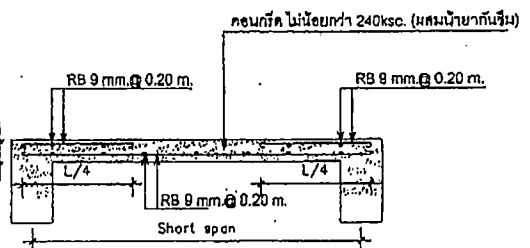
S1(ด้านต้น) มาตราส่วน 1:20
