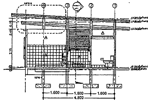
Section 4 มาตราส่วน 1:100
