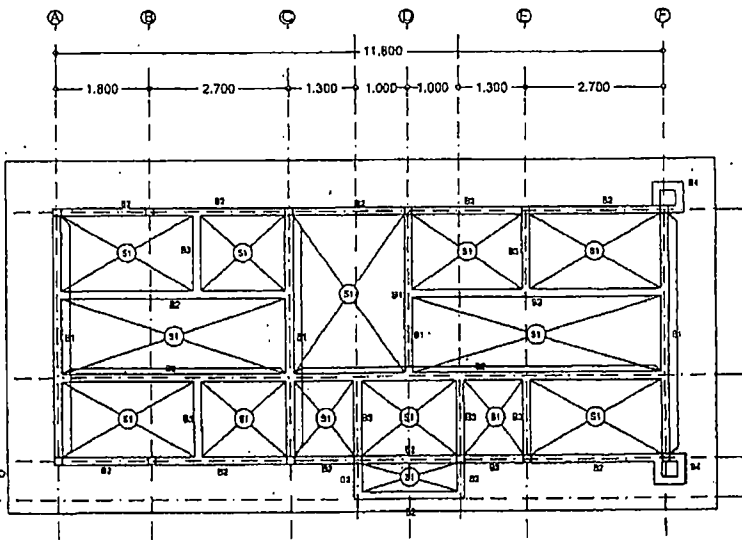
แปลนฐาน ค.ส.ล. มาตราส่วน 1:100
