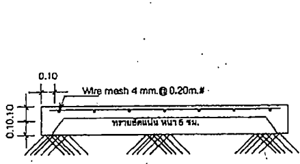
GS มาตราส่วน 1:20
