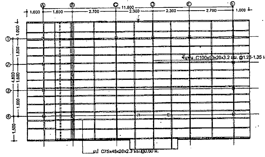
แปลนโครงสร้างหลังคา มาตราส่วน 1:50
