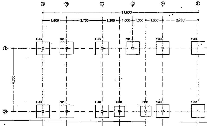
แปลนฐานราก เสา ค.ส.ล. มาตราส่วน 1:100
