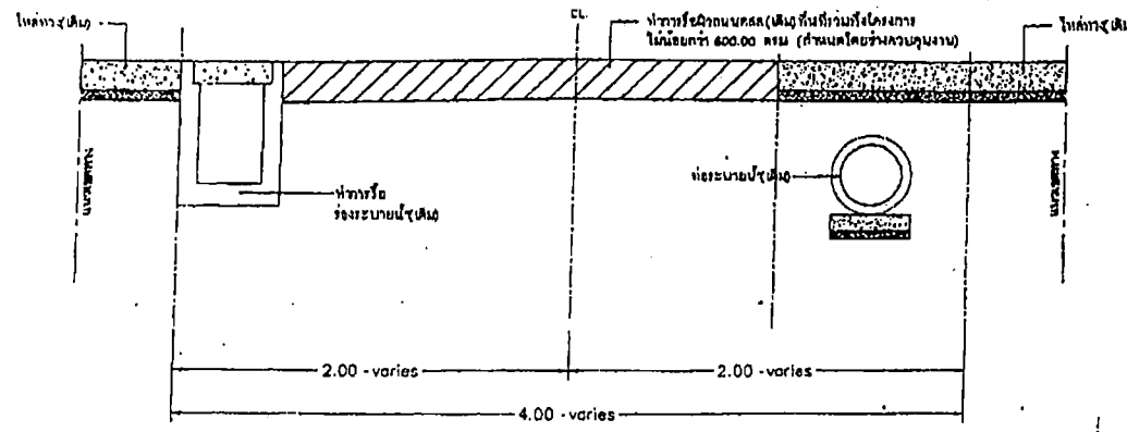
รูปตัด 2 (เก่า) NOT TO SCALE
