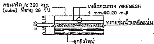
ขยายถนน ค.ส.ล.และโหลทาง ค.ส.ล.หนาไม่น้อยกว่า 0.15 ม. NOT TO SCALE
