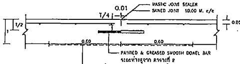
รูปตัดตามขวางที่วางตัวจากราว คสล.
