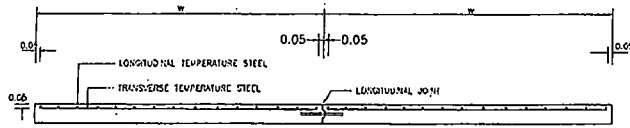
รูปตัดตามขวางที่วางตัวจากราว คสล.
