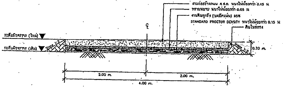
รูปตัด 1 NOT TO SCALE
