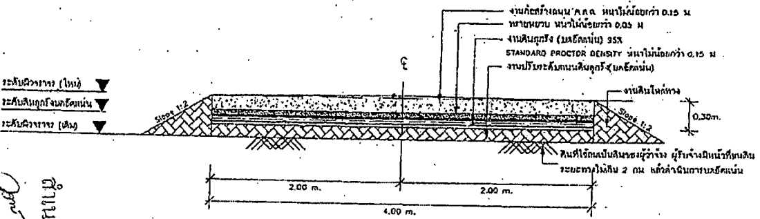
รูปตัด 2 NOT TO SCALE
